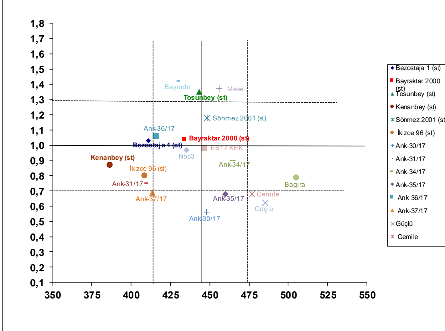
Grafik 2. Orta Anadolu Bölgesi Kuruda Ekmeklik Buğday-2 Stabilité Grafığı
